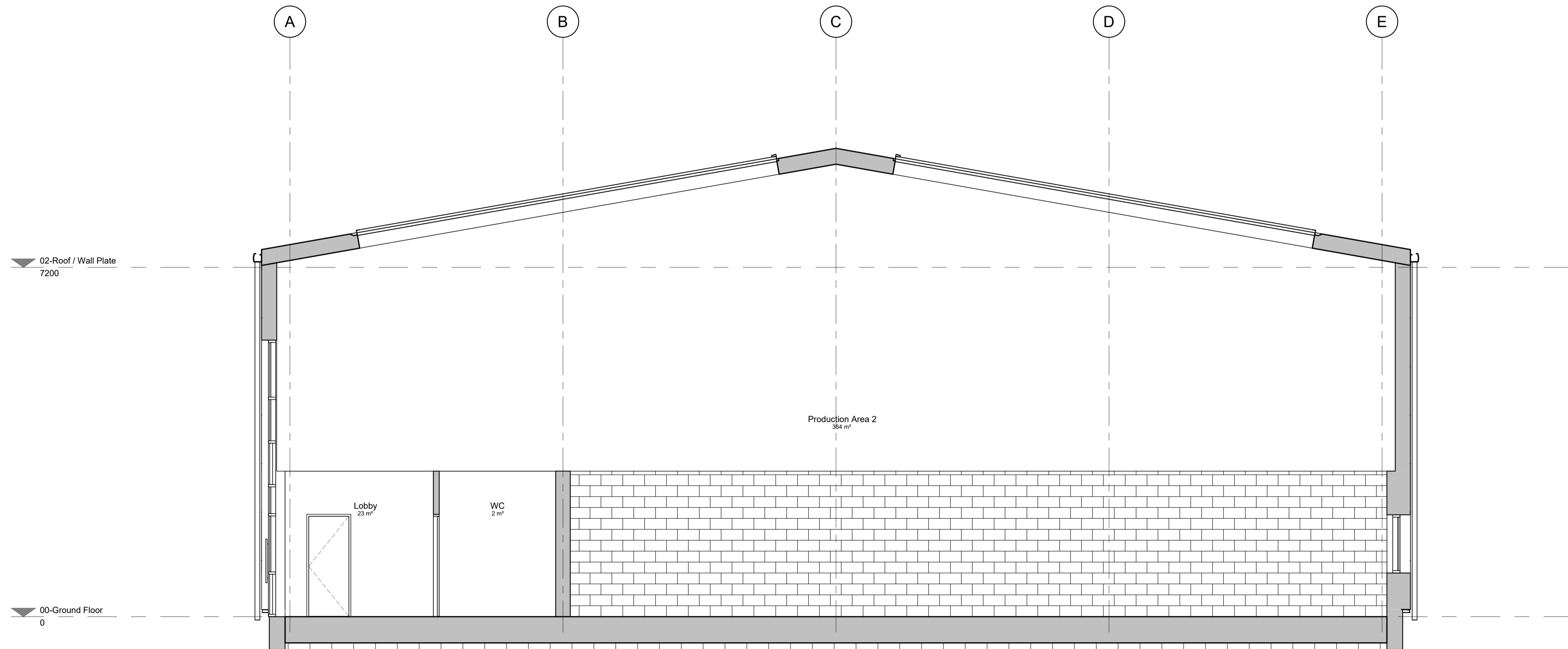
1 Section 1 1 : 50
