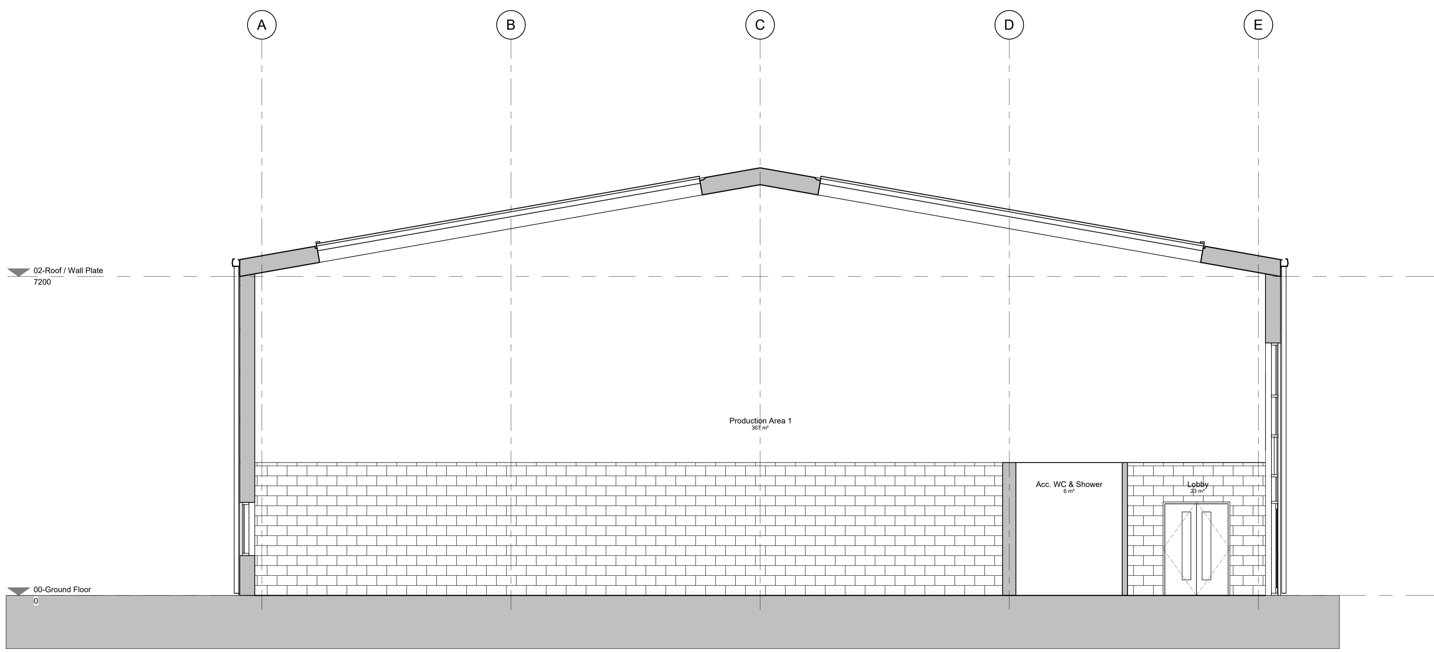
1 Section 1 1 : 50
