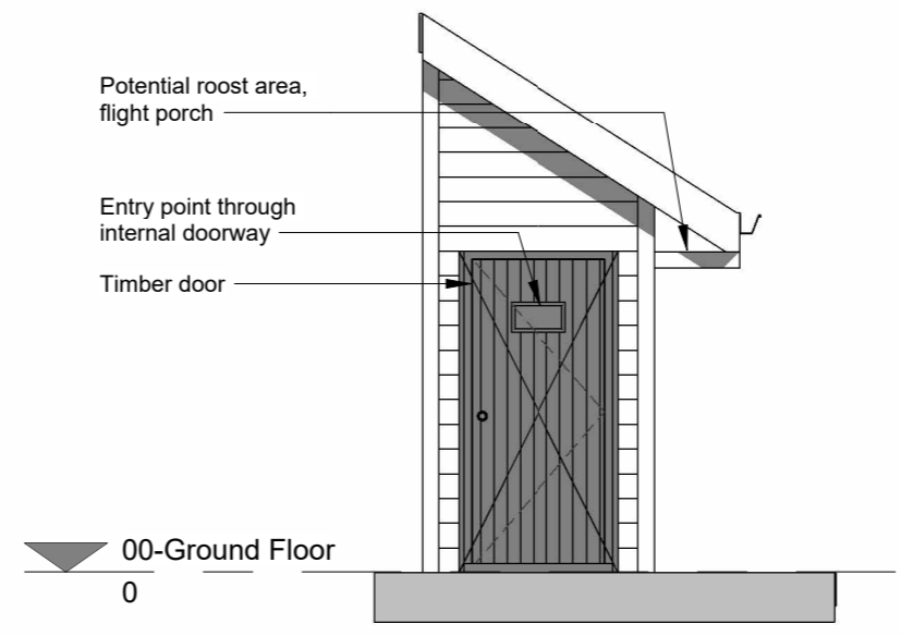
2 Side Elevation - Door 1 : 50
